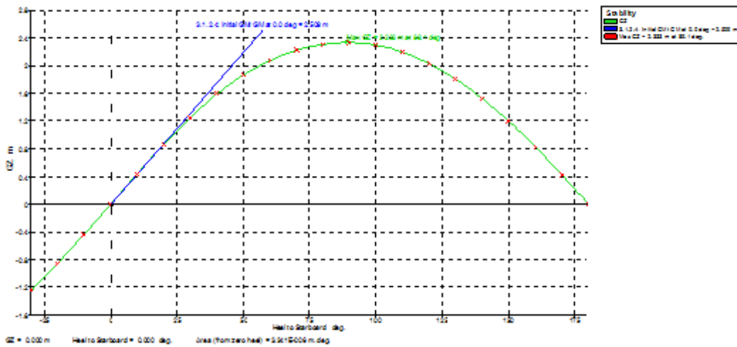
Gambar 3. Kurva GZ pada Ketinggian Gelombang 2 m.
