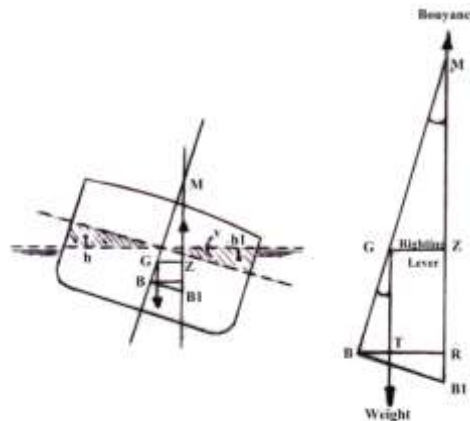
Gambar 1. Stabilitas pada Sudut Inklinasi yang Besar
