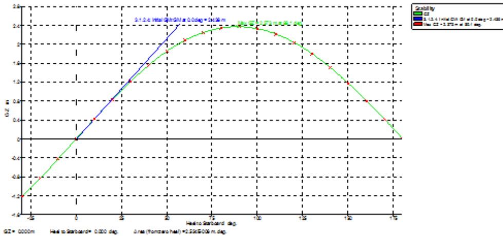
Gambar 5. Kurva GZ pada Ketinggian Gelombang 4 m.
