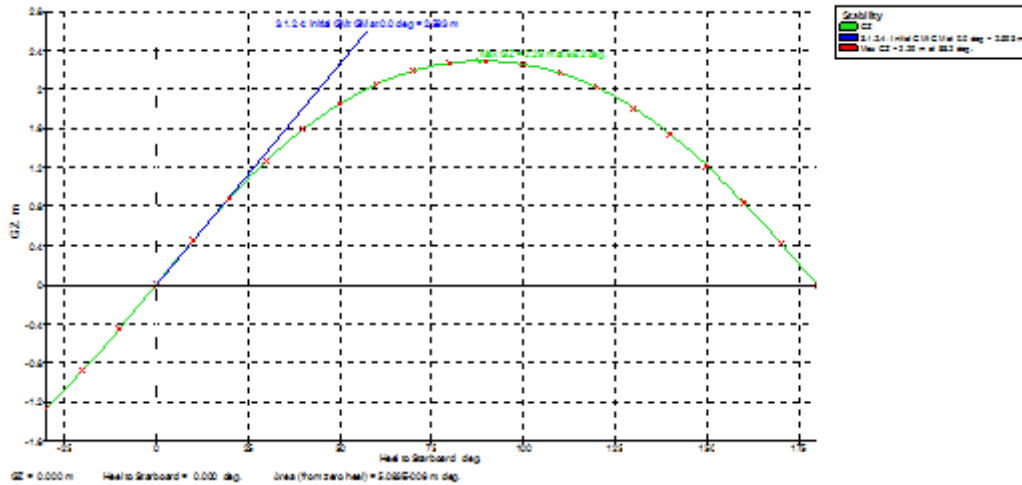
Gambar 2. Kurva GZ pada Ketinggian Gelombang 1 m.
