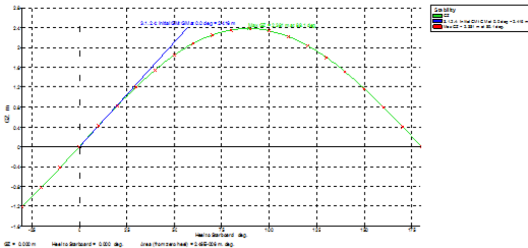
Gambar 6. Kurva GZ pada Ketinggian Gelombang 6 m.
