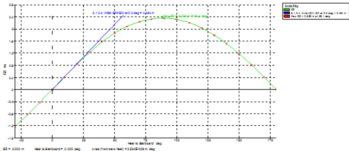
Gambar 4. Kurva GZ pada Ketinggian Gelombang 3 m.
