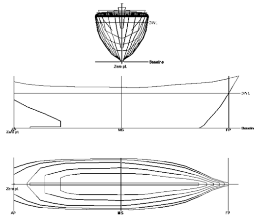
Gambar 3. Lines plan kapal purse seine di Kabupaten Tanah Laut
