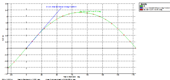
Gambar 4. Kurva GZ kapal purse seine di Kabupaten Tanah Laut
