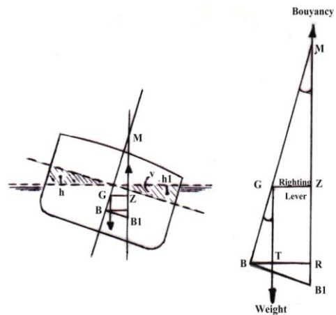
Gambar 2. Stabilitas pada Sudut Inklinsi yang Besar
