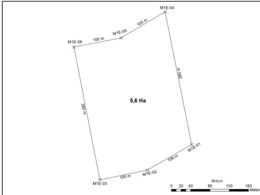
Gambar-3. Jarak antar Lubang Bor
