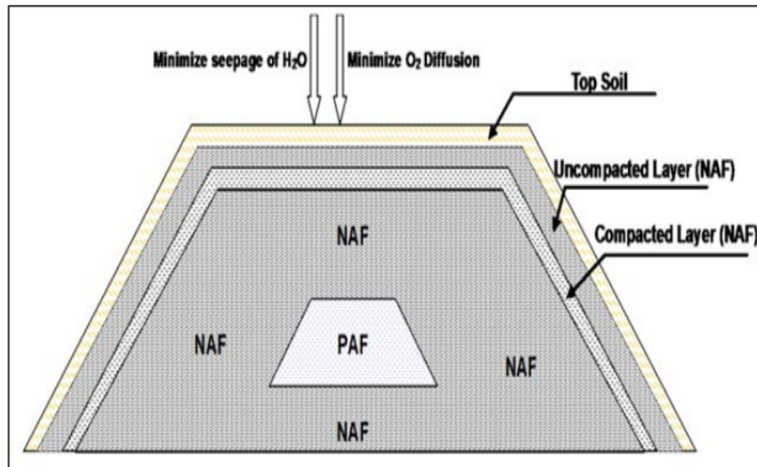
Gambar-5. Metode Enkapsulasi material PAF dan NAF
