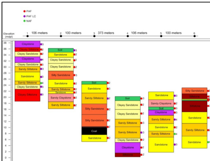
Gambar-4. Litologi Penggolongan Material PAF dan NAF
