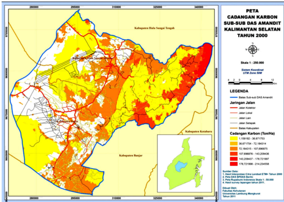
Gambar 2. Peta cadangan karbon Sub-sub DAS Amandit tahun 2000
