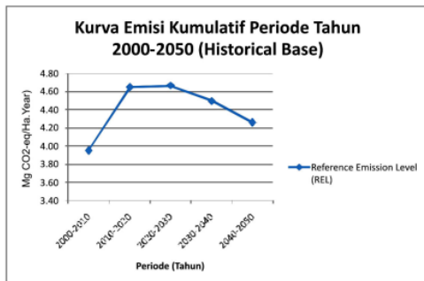
Gambar 5. Kurva emisi kumulatif periode tahun 2000-2050 (Historical Base)
