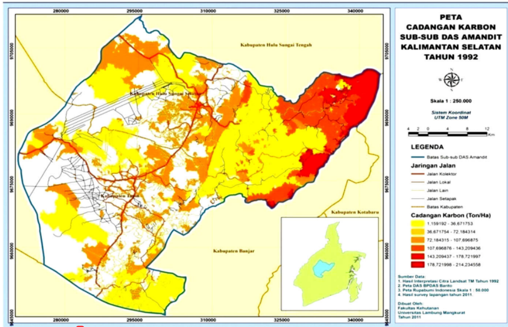
Gambar 1. Peta cadangan karbon Sub-sub DAS Amandit tahun 1992
