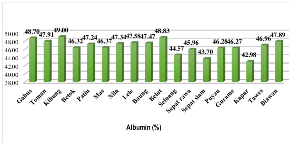
Gambar 1. Diagram profil albumin ikan konsumsi
