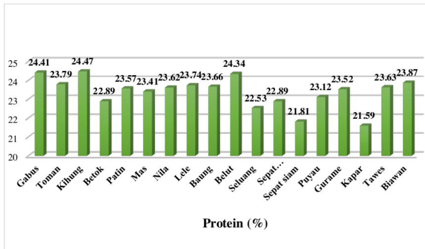
Gambar 2. Diagram profil protein ikan konsumsi
