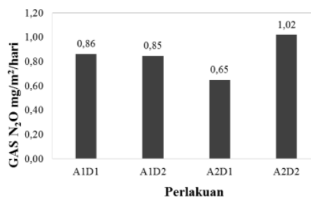
Gambar 2. Pengaruh pemberian berbagai kombinasi bahan amelioran dan pupuk terhadap nilai Gas N 2 O (mg/m 2 /hari) pada tanah gambut
