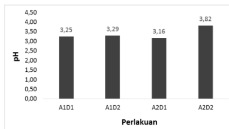
Gambar 3. Pengaruh pemberian berbagai kombinasi bahan amelioran dan pupuk terhadap nilai pH pada tanah gambut.
