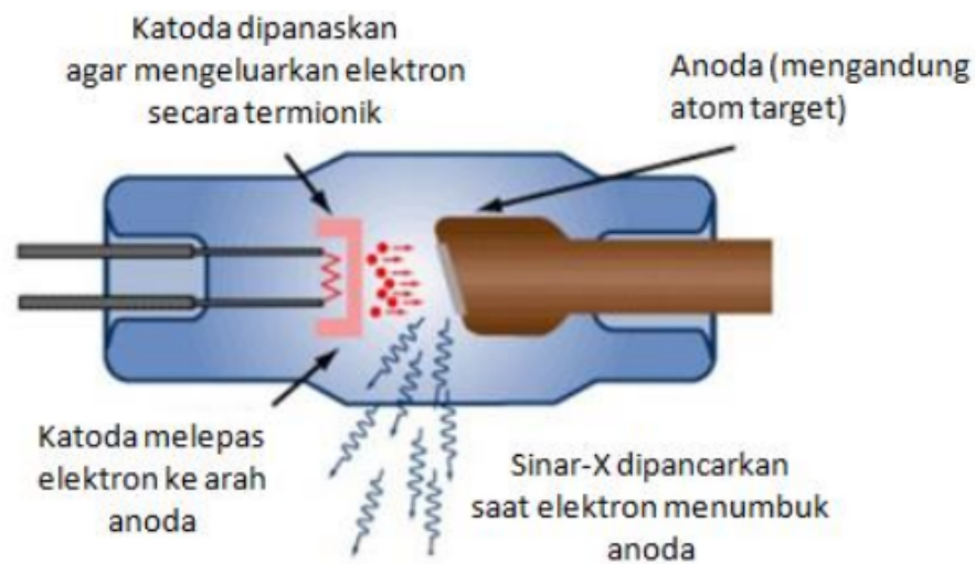
Gambar 1. 1 Pesawat sinar X
