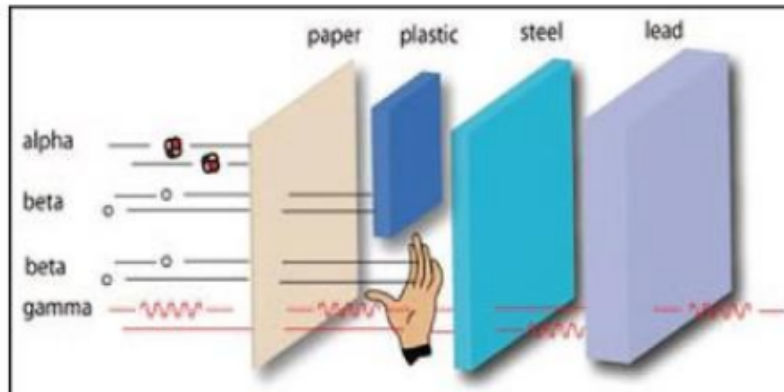
Gambar 2. 1 Perbandingan tingkat penetrasi dari sinar radiasi terionisasi (Zakariya dan Kahn, 2014).
