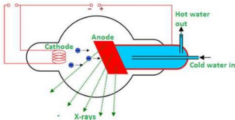
Gambar 2. 2 Proses terbentuknya sinar-X (Prabhu dkk, 2020)
