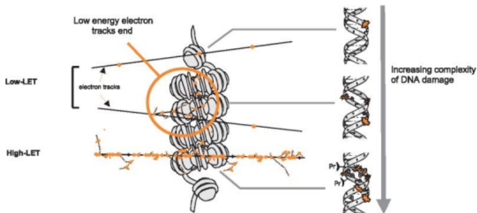
Gambar 1. 2 Proses ionisasi disertai kerusakan DNA oleh LET tinggi dan LET rendah (IARC 2014).
