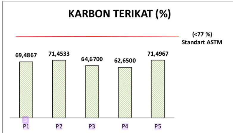
Gambar 5. Grafik Rata-rata Nilai Karbon Terikat (%)
