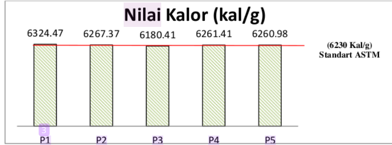
Gambar 9. Grafik Rata-rata Nilai Kalor (kal/g)
