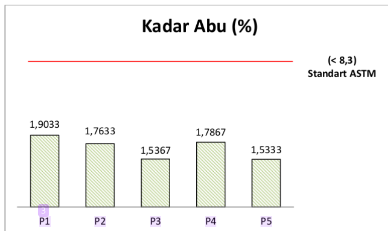
Gambar 3. Grafik Rata-rata Nilai Kadar Abu (%)
