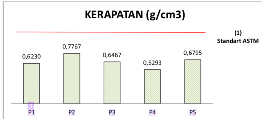
Gambar 2. Grafik Rata-rata Kerapatan (g/cm 3 )
