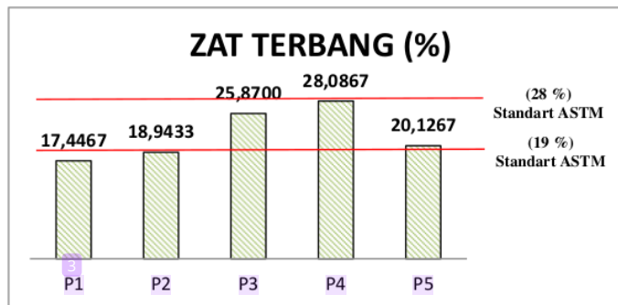
Gambar 4. Grafik Rata-rata Nilai Zat Terbang (%)
