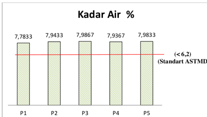
Gambar 1. Grafik Rata-rata Kadar Air (%)
