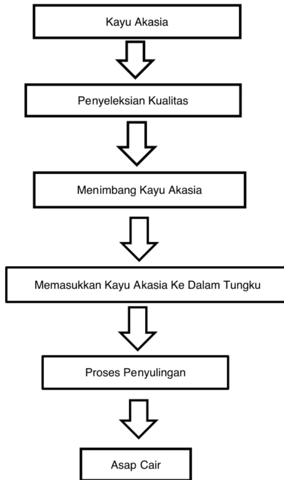
Gambar 1. Skema Pembuatan Asap Cair
