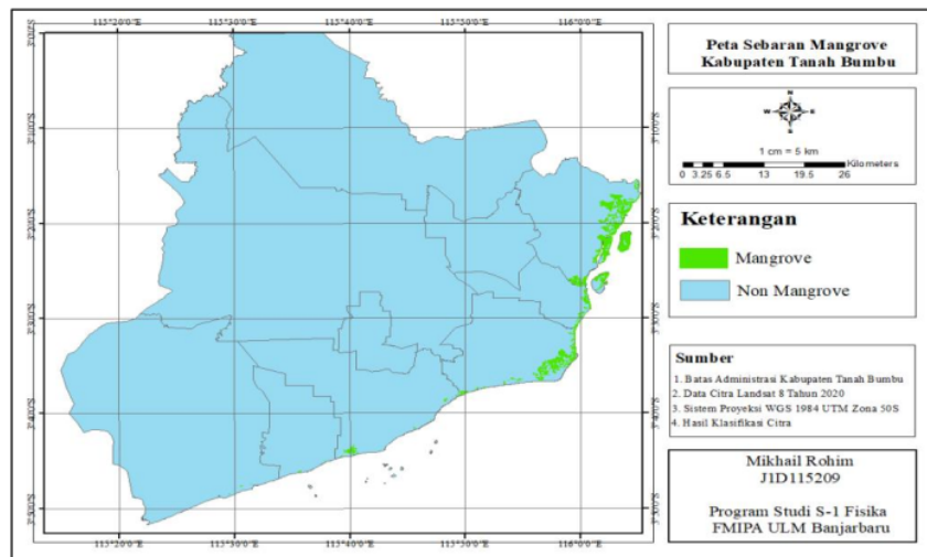
Gambar 2 Hasil sebaran Mangrove di Kabupaten Tanah Bumbu .
