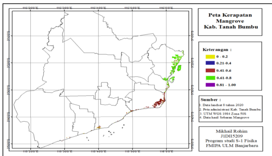
Gambar 2 Hasil Kerapatan dengan Menggunakan Metode NDVI.
