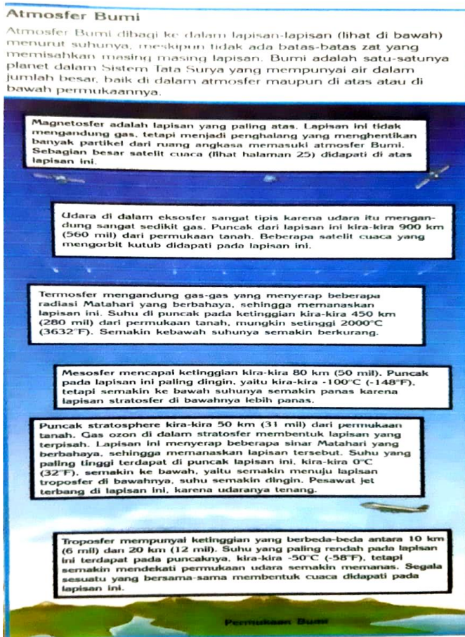
Gambar 1. Bentuk lapisan atmosfer bumi
