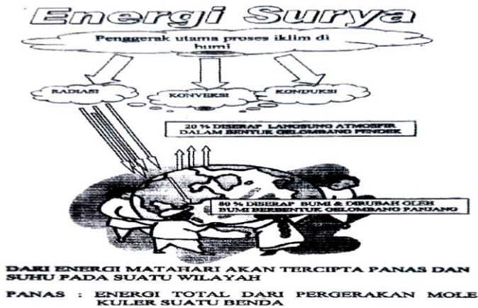
Gambar 3. Pancaran Energi Matahari
