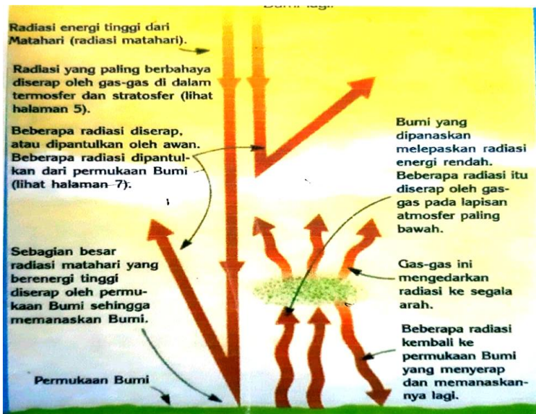
Gambar 4. Penyimpangan Penghilangan Radiasi Matahari Yang Melalui Atmosfer
