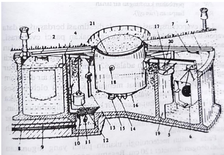
Gambar 18. Lysimeter untuk mengukur laju evapotranspirasi
