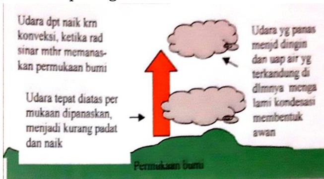
Gambar 15. Penaikan udara karena pemanasan dan pendinginan udara
