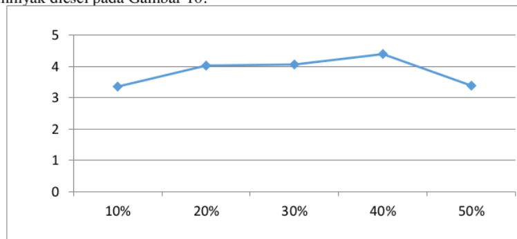
Gambar 10. Grafik pengaruh variasi campuran crude palm oil dan minyak diesel terhadap burning rate
