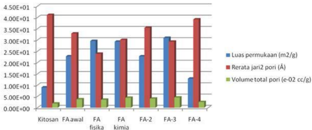
Gambar 2. Profil perubahan luas permukaan, rerata jari2 pori, dan volume total pori dari bahan baku dan pellet komposit yang terbentuk.
