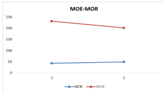
Gambar 2. Hasil Pengujian MOE-MOR
