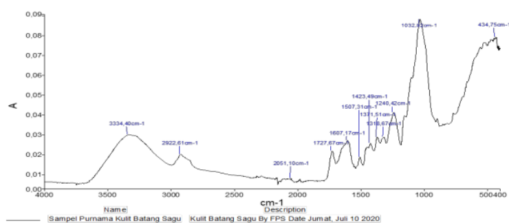
Gambar 1. Spektrum gelombang kulit batang sagu
