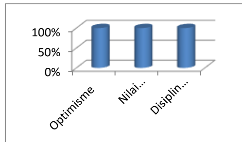
Gambar 1. Diagram Kategori Kelompok Skor X1, X2, Y
