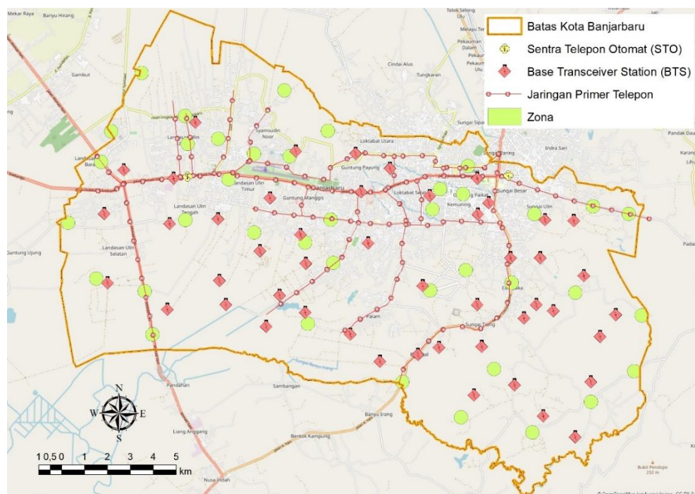
Gambar 4.15. Jaringan telekomunikasi Kota Banjarbaru
