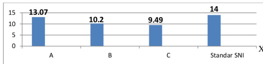
Gambar 1. Diagram Kadar air papan komposit
