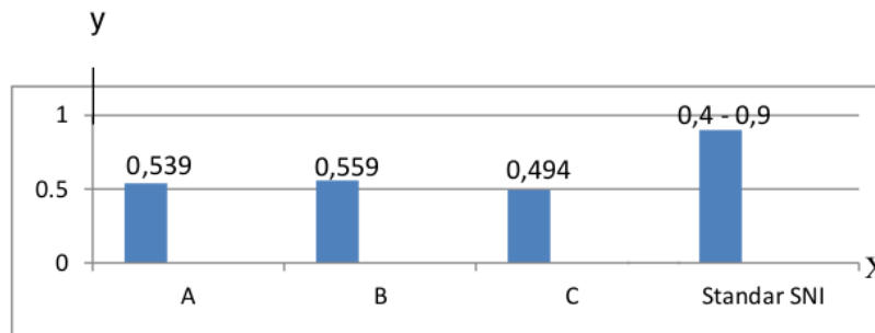
Gambar 2. Diagram Kerapatan papan komposit
