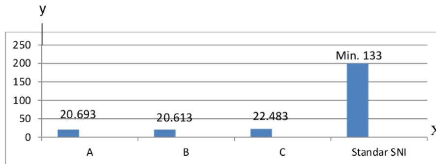
Gambar 4. Diagram Keteguhan patah papan komposit
