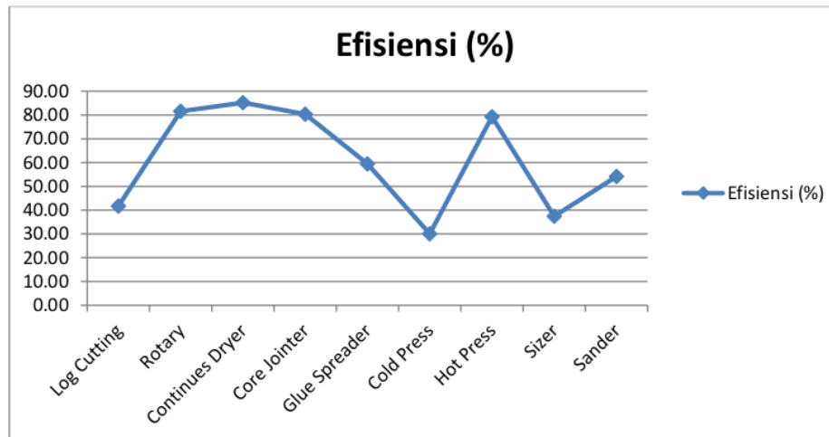
Gambar 2. Grafik Nilai Efisiensi Penggunaan Mesin
