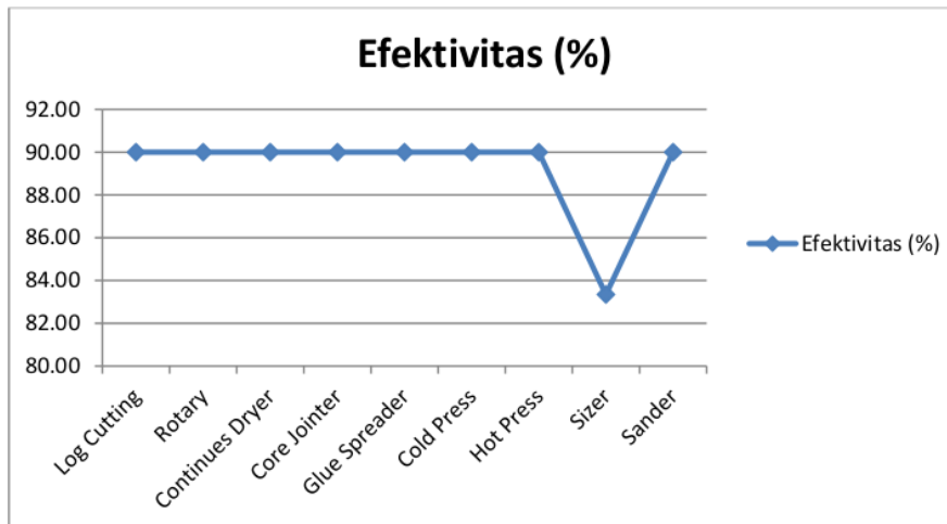
Gambar 1. Nilai Efektifitas Penggunaan Mesin
