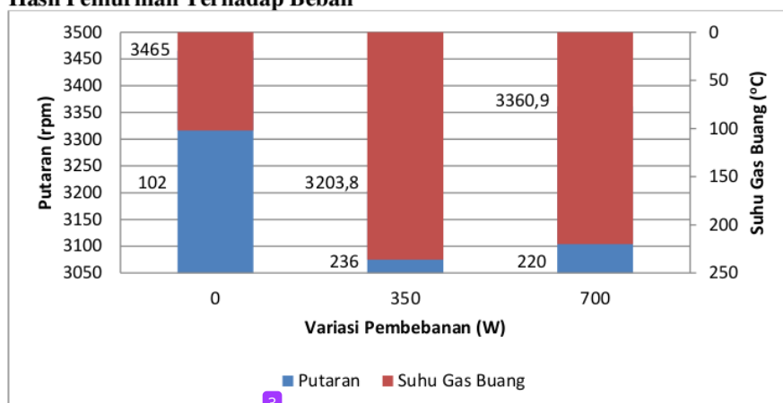
3 Gambar 7. Hubungan unjuk kerja generator-set menggunakan bahan bakar biogas hasil pemurnian terhadap penambahan beban
