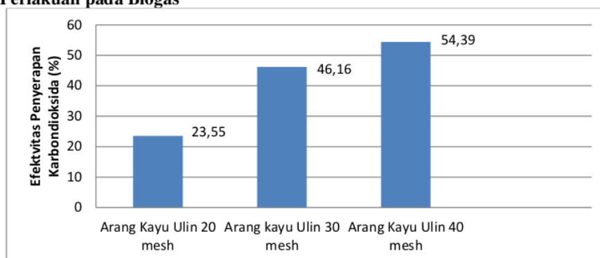
Gambar 4. Hubungan efektivitas penyerapan CO 2 pada pemurnian biogas dengan perlakuan pada biogas
