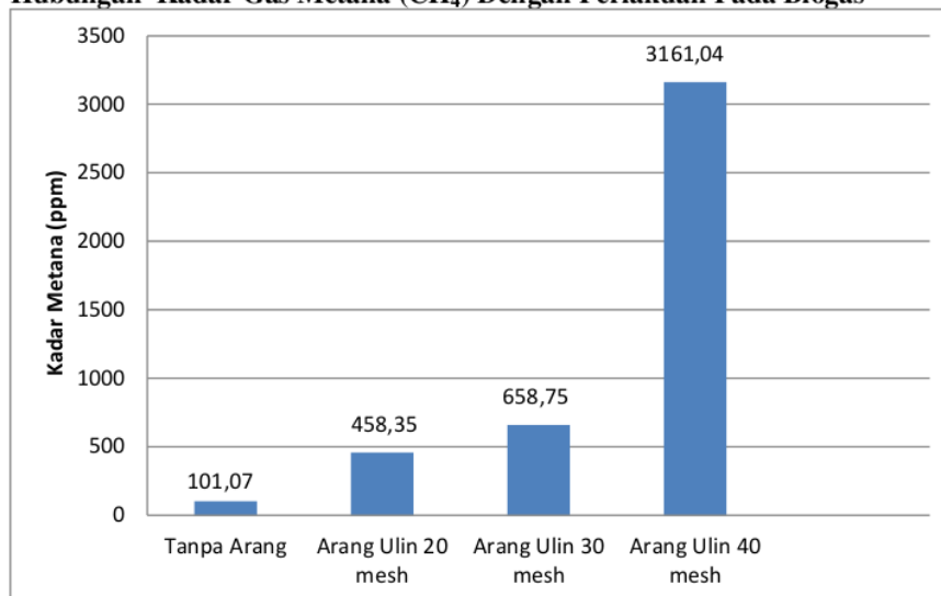
Gambar 3. Hubungan Kadar Gas Metana Dengan Perlakuan Pada Biogas
