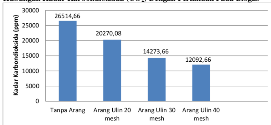
Gambar 2. Hubungan Kadar Karbondioksida Dengan Perlakuan Pada Biogas
