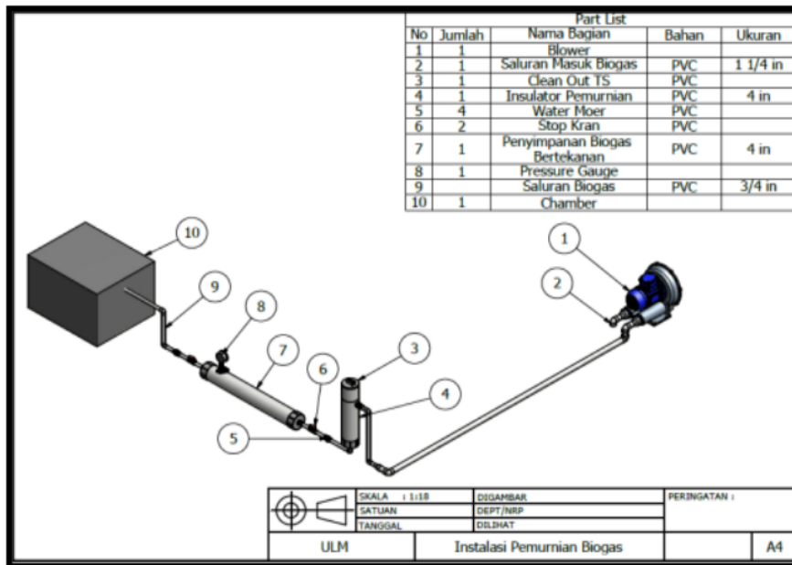
Gambar 1. Skema Alat Pemurnian Biogas
