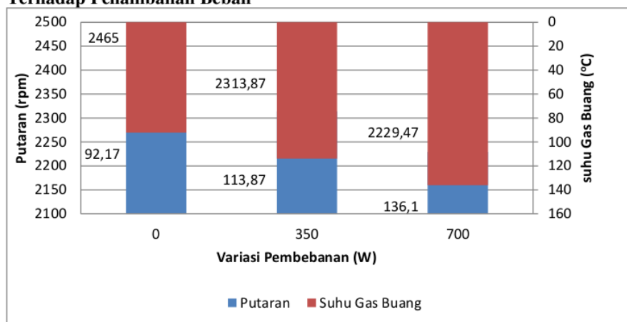
Gambar 6. Hubungan unjuk kerja generator-set menggunakan bahan bakar pertalite terhadap penambahan pembebanan
