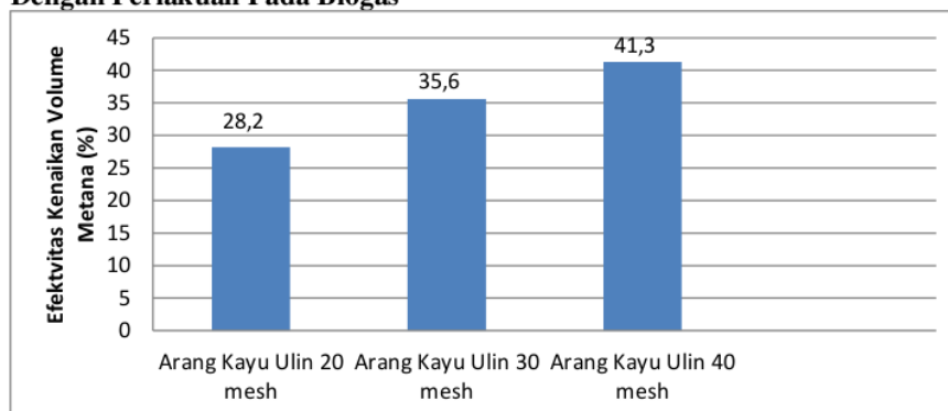
Gambar 5. Hubungan kenaikan volume CH 4 pada pemurnian biogas dengan perlakuan pada biogas
