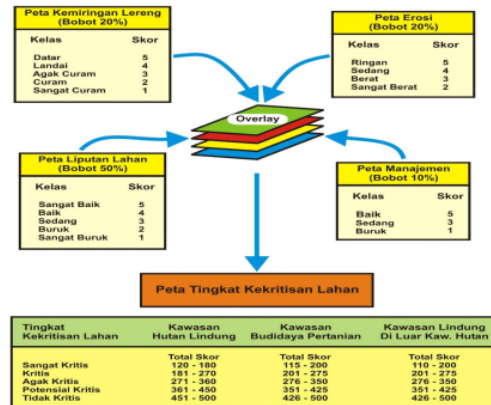
Gambar 2. Diagram alir penentuan tingkat kekritisitas lahan
