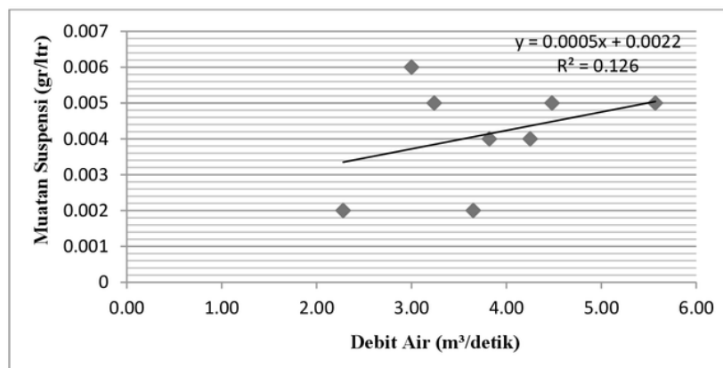
Gambar 10. Grafik hubungan antara muatan suspensi dengan debit air bagian Hulu
