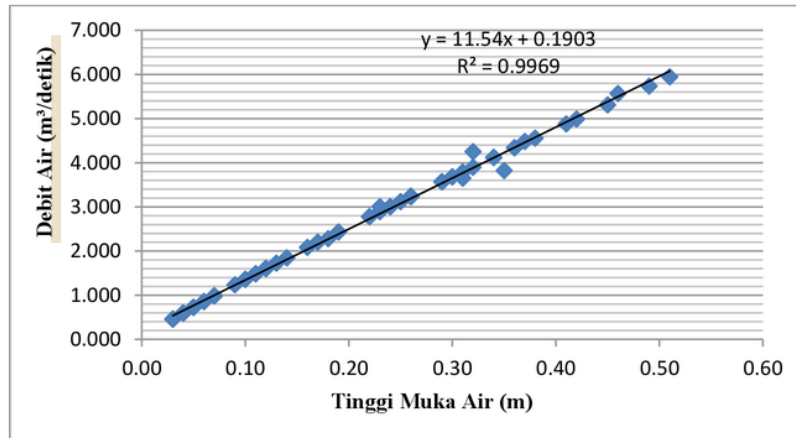
Gambar 4. Grafik hubungan antara TMA dengan debit air bagian Hulu
