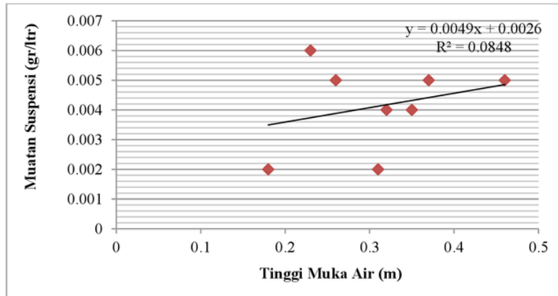
Gambar 7. Grafik hubungan antara Muatan Suspensi dengan TMA bagian Hulu
