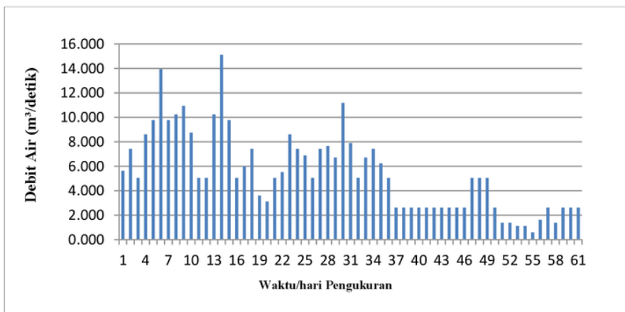
Gambar 2. Diagram hasil pengukuran debit air bagian Tengah
