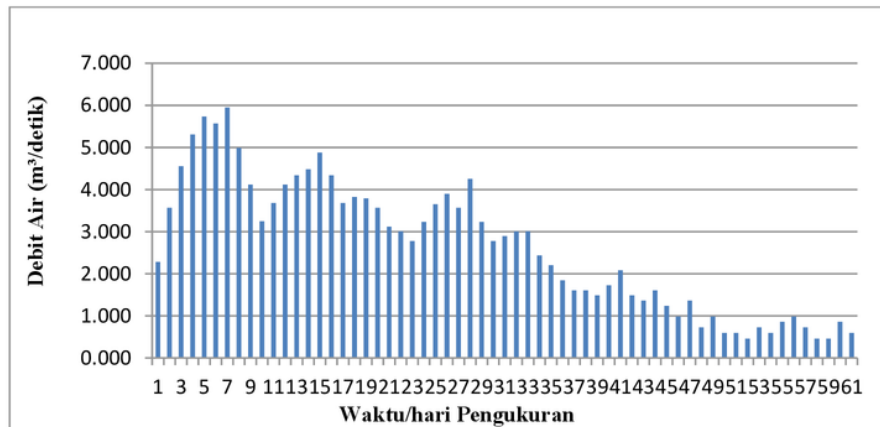
Gambar 1. Diagram hasil pengukuran debit air bagian Hulu
