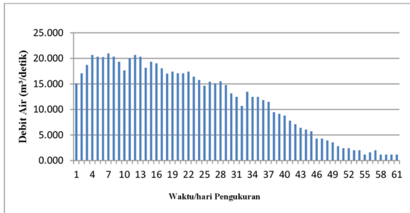
Gambar 3. Diagram hasil pengukuran debit air bagian Hilir
