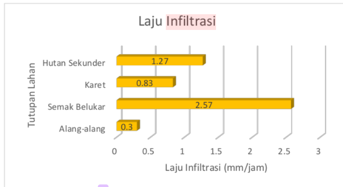
Gambar 2. Laju Infiltrasi Pada Berbagai Tutupan Lahan
