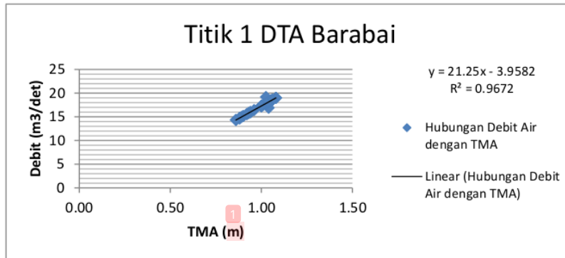
Gambar 4. Grafik hubungan tinggi muka air dengan debit air titik 1
