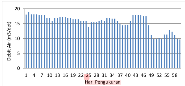
Gambar 2. Diagram hasil pengukuran debit air titik 2
