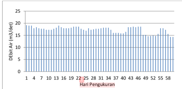
Gambar 1. Diagram hasil pengukuran debit air titik 1
