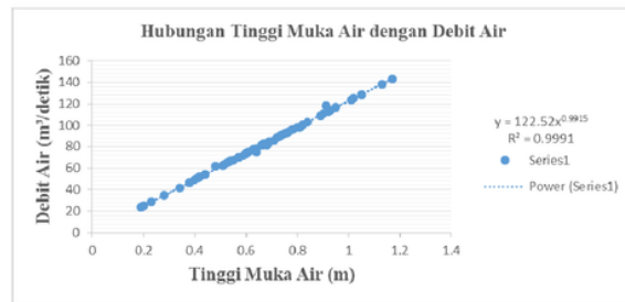
Gambar 6. Grafik Hubung Tinggi Muka Air dengan Debit Air Bagian Hilir
