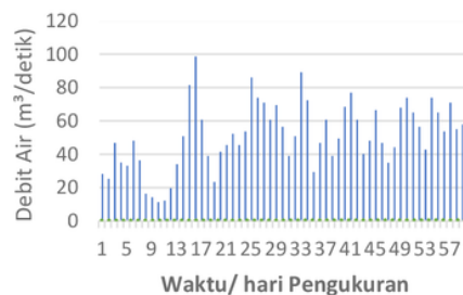
Gambar 3. Diagram Hasil Pengukuran Debit Air Bagian Hulu
