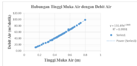
Gambar 5. Grafik Hubung Tinggi Muka Air dengan Debit Air Bagian Hulu
