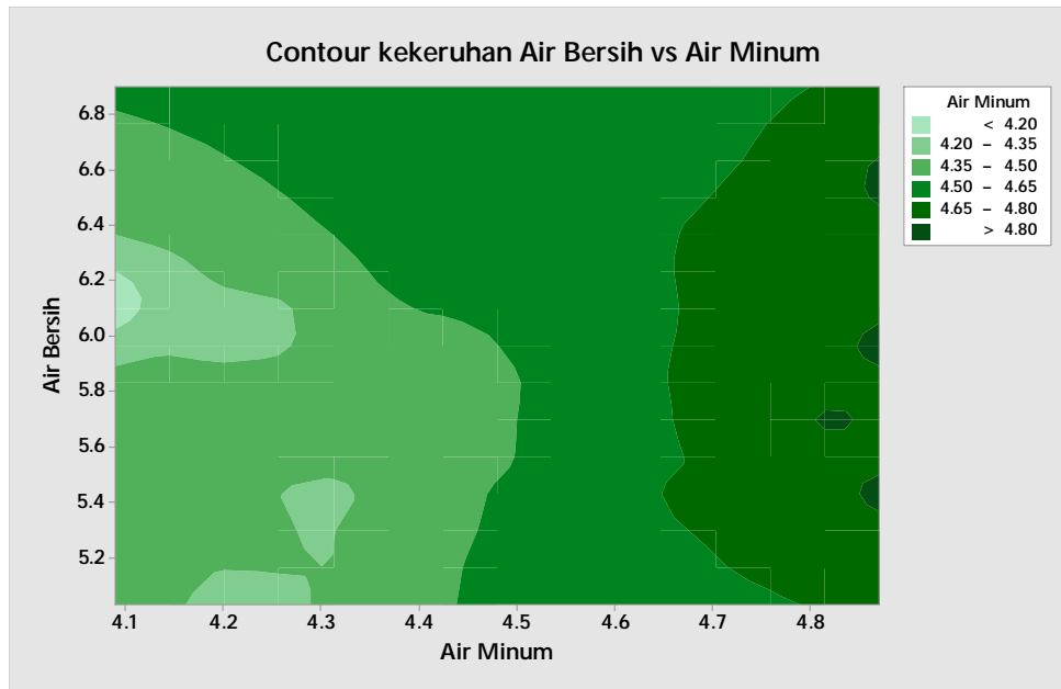
Gambar 5.2 Plot Contour kekeruhan air baku dan air proses pencampuran
