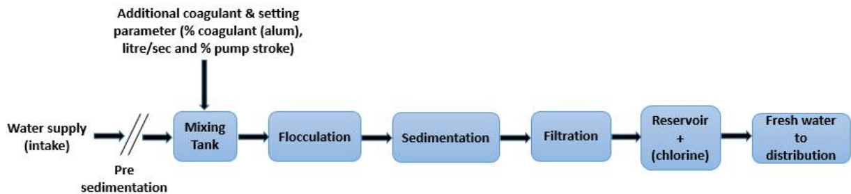
Gambar 2.1 Proses produksi air bersih/minum
