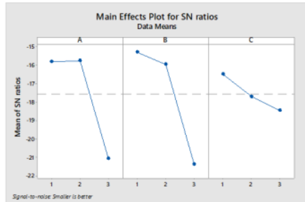
Gambar 2. Grafik respon S/N ratio kekasaran permukaan
