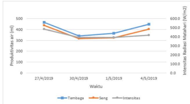
Gambar 7. Grafik Perbandingan Produktivitas Air
