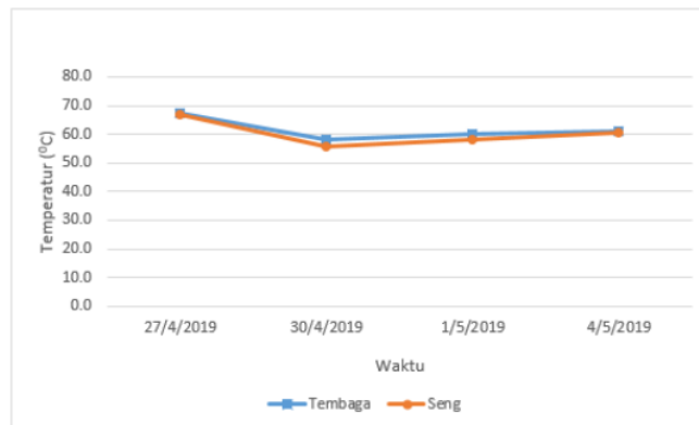
Gambar 10. Grafik Perbandingan Temperatur Air Pada Solar Distillation Dengan Absorber Tembaga Dan Seng
