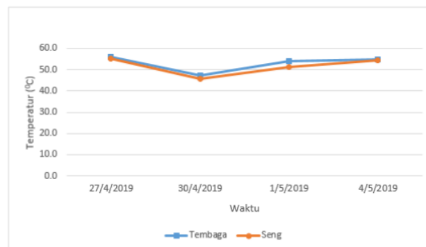
Gambar 12. Grafik Perbandingan Temperatur Kaca Pada Solar Distillation Dengan Absorber Tembaga Dan Seng
