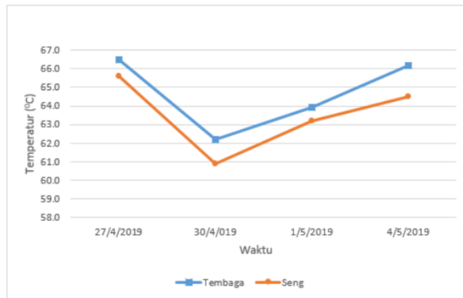
Gambar 9. Grafik Perbandingan Temperatur Plat Pada Solar Distillation Dengan Absorber Tembaga Dan Seng
