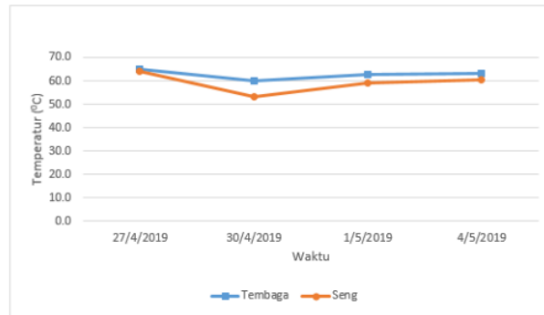
Gambar 11. Grafik Perbandingan Temperatur Ruang Basin Pada Solar Distillation Dengan Absorber Tembaga Dan Seng
