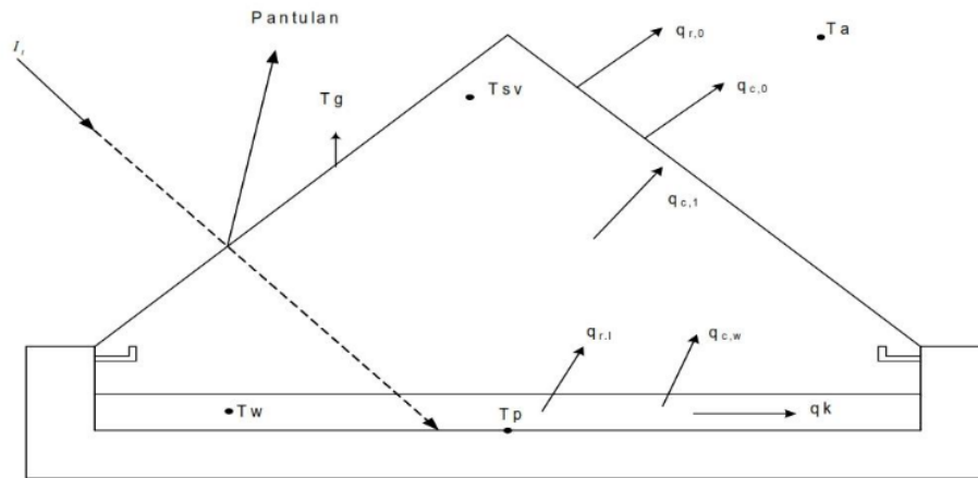
Gambar 3. Diagram Alir Energi
