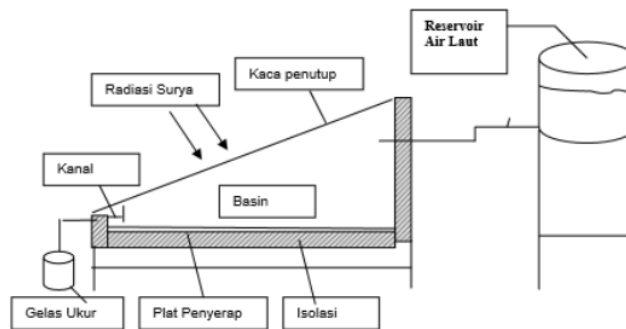
Gambar 2. Solar Distillation Dengan Satu Permukaan Kaca
