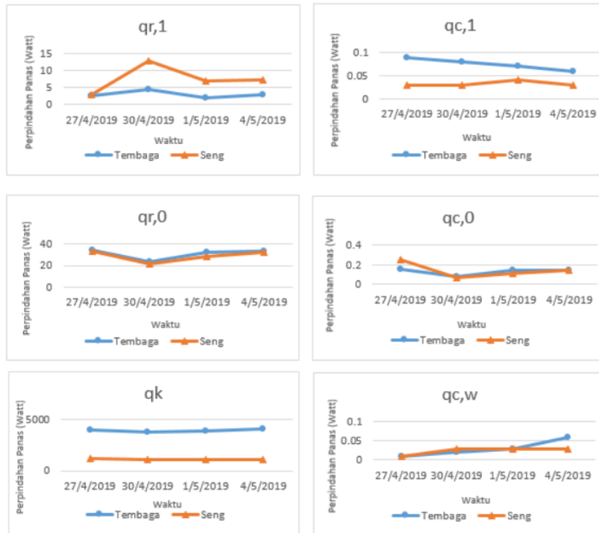
Gambar 8. Perpindahan Panas Pada Solar Distillation
