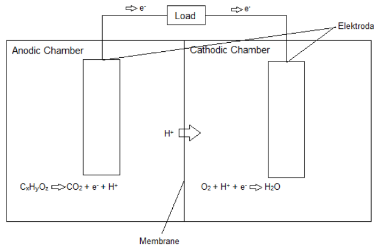
Gambar 3. Prinsip kerja MFC
