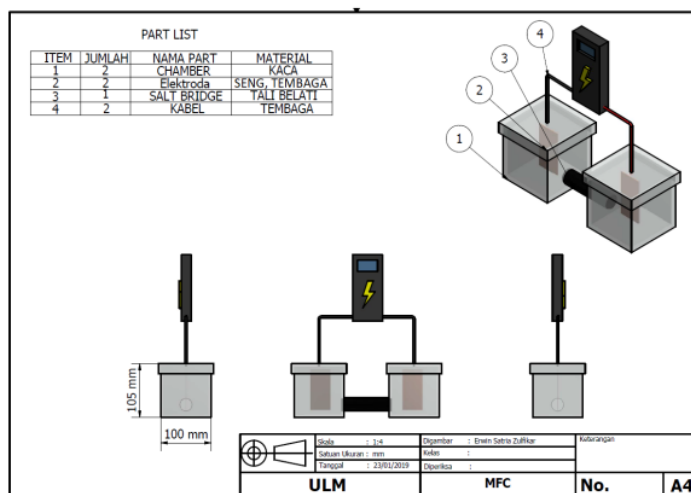
Gambar 5. Desain MFC
