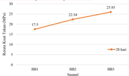
Gambar 2. Hasil kuat tekan sampel blok perkerasan
