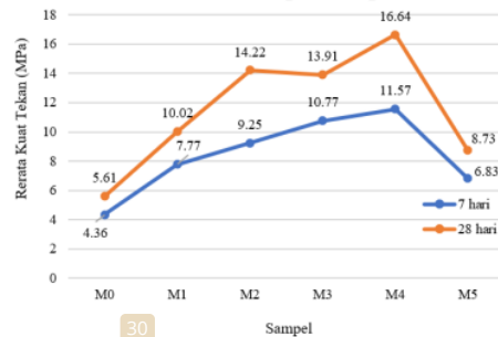
Gambar 1. Hasil kuat tekan sampel mortar
