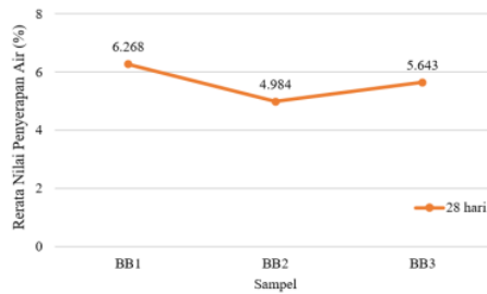
Gambar 3. Hasil Pengujian Penyerapan Air
