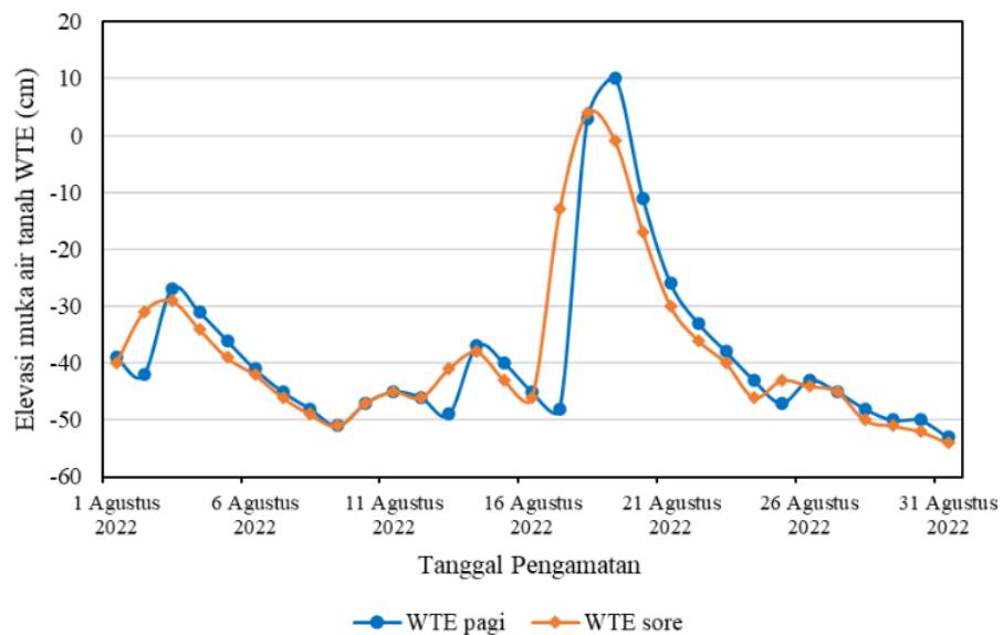
8 Gambar 8 Grafik Fluktuasi Muka Air Tanah (WTE) selama bulan Agustus di lokasi 2
