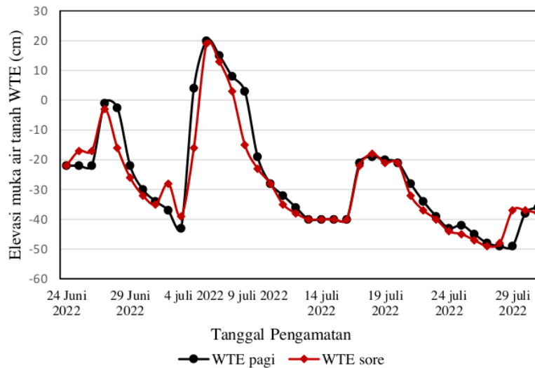
Gambar 6 Grafik Fluktuasi Muka Air Tanah (WTE) selama bulan Juli di lokasi 2
