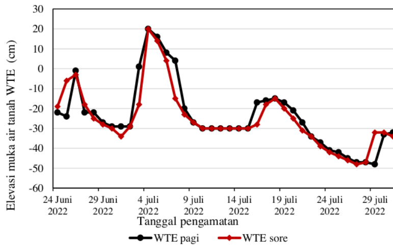
Gambar 5 Grafik Fluktuasi Muka Air Tanah (WTE) selama bulan Juli di lokasi 1
