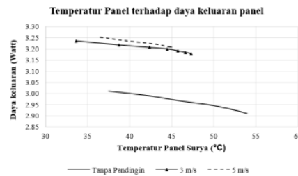
Gambar 5. Efek Temperatur Panel Terhadap Daya Keluaran Panel Surya
