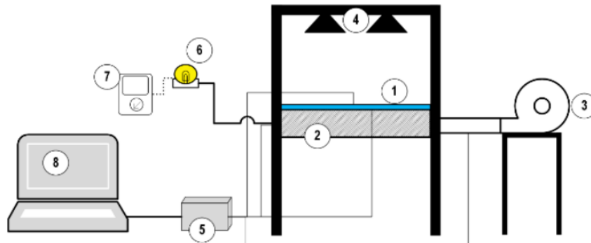
Gambar 1. Rangkaian Skematik Eksperimen
