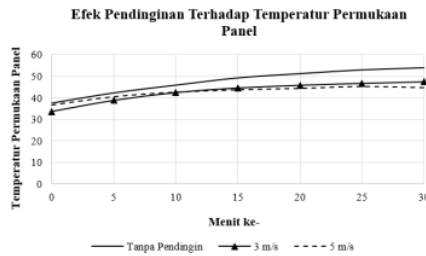
Gambar 4. Efek Pendingin Terhadap Temperatur Permukaan Panel
