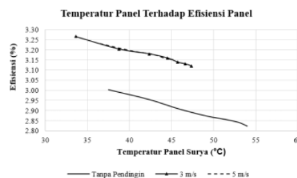
Gambar 6. Efek Temperatur Panel Terhadap Efisiensi Panel Surya
