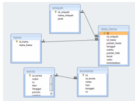
Gambar 4 ERD Sistem
