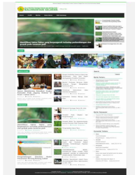
Gambar 6 Form Utama
