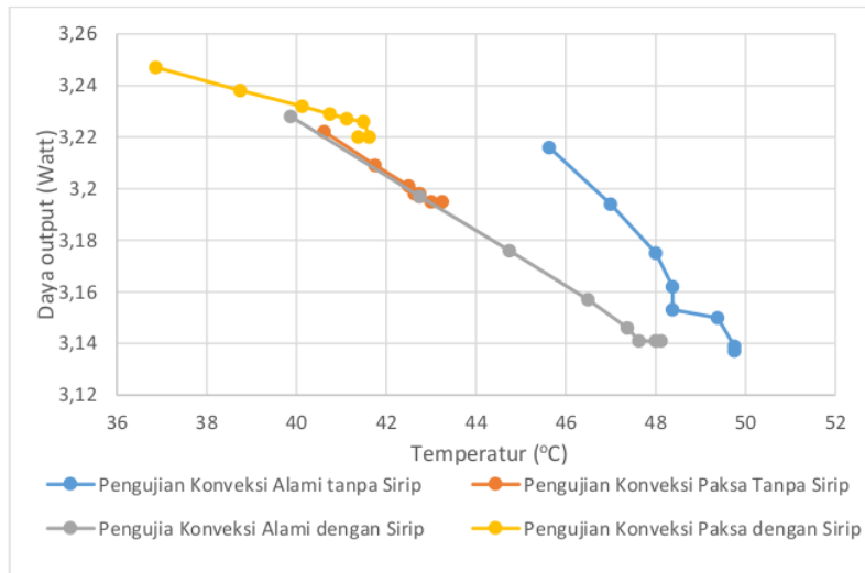
Gambar 5. Grafik Pengaruh Temperatur Terhadap Daya Output
