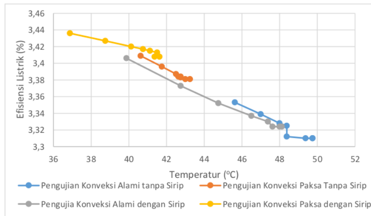
Gambar 6. Grafik Pengaruh Temperatur Terhadap Efisiensi Listrik
