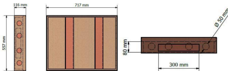
Gambar 2. Kotak Pendingin
