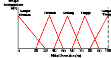
Gambar 6 Fungsi Keanggotaan Output
