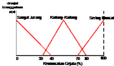
Gambar 4 Fungsi Keanggotaan Input 1
