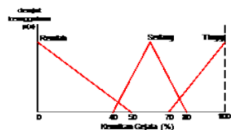
Gambar 5 Fungsi Keanggotaan Input 2
