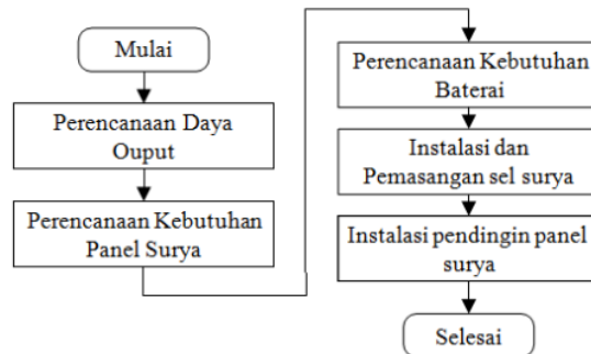
Gambar 2. Tahapan Perencanaan Teknologi Sel Surya Berpendingin Air
