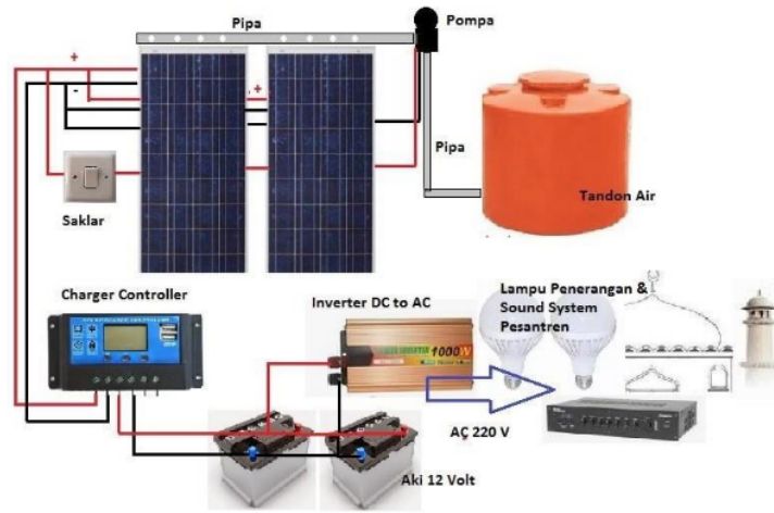
Gambar 3. Teknologi Sel Surya Berpendingin Air
