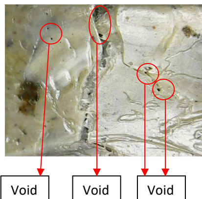
Gambar 20. Foto Makro Hasil Patahan Spesimen Uji Bending (B1.1)
