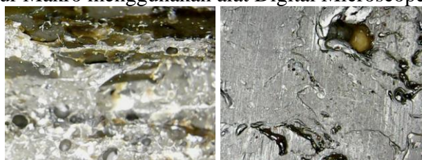
Gambar 4. Foto Makro Patahan dan Permukaan Spesimen A1.2 30% Oli Bekas + 70% HDPE dan PET (50%:50%)
