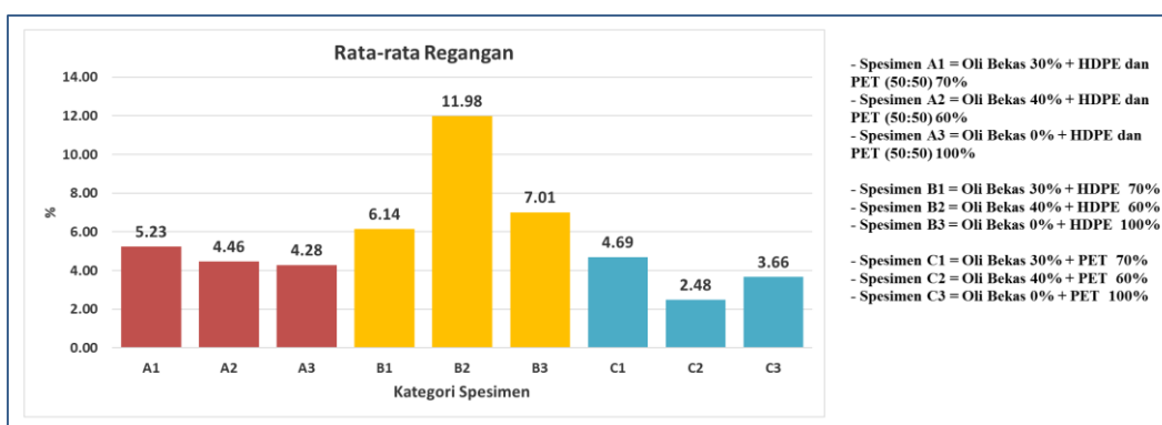
Gambar 14. Grafik Rata-Rata Regangan Spesimen Uji Tarik
