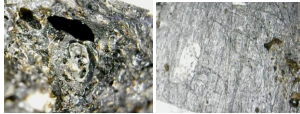
Gambar 6. Foto Makro Patahan dan Permukaan Spesimen A3.2 0% Oli Bekas + 100% HDPE dan PET (50%:50%)
