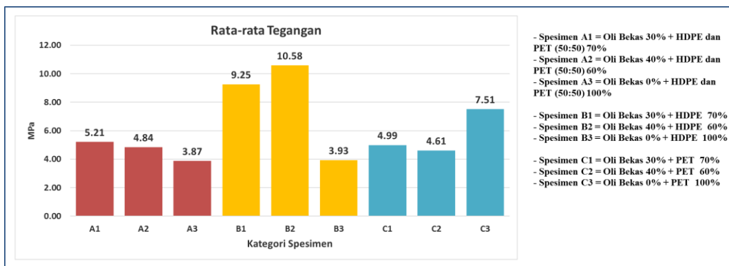
Gambar 13. Grafik Rata-Rata Tegangan Spesimen Uji Tarik
