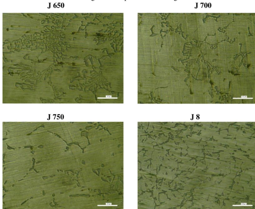
Gambar 17. Hasil Pengujian Struktur Mikro Wajan Jawa
