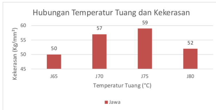
Gambar 16. Hasil Pengujian Kekerasan Wajan Jawa
