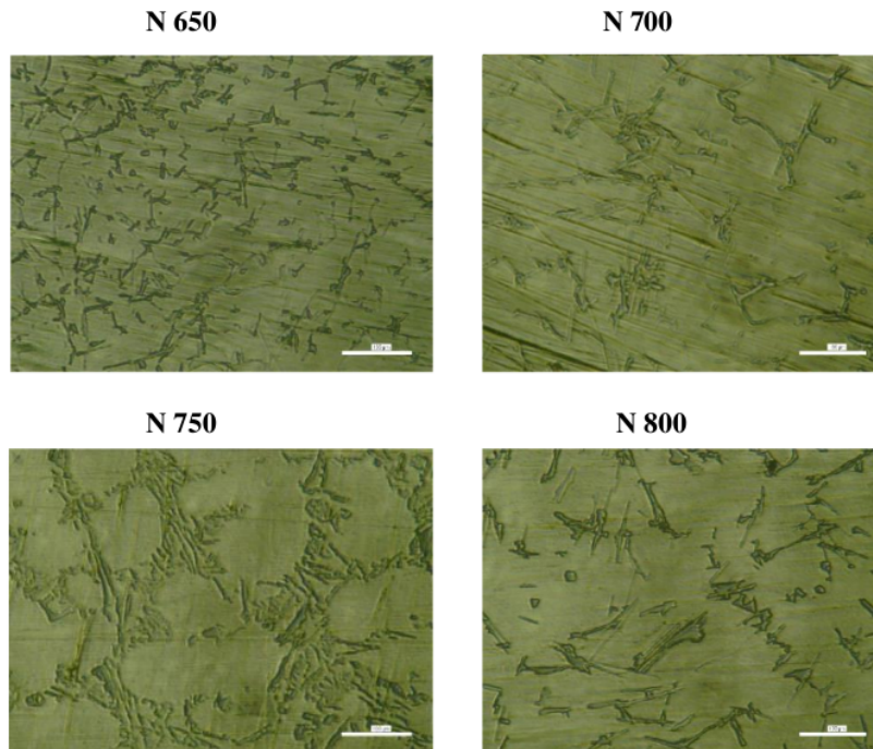
Gambar 14. Hasil Pengujian Struktur Mikro Wajan Nagara
