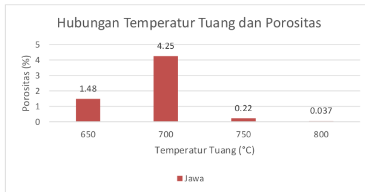
Gambar 15. Hasil Pengujian Porositas Wajan Jawa
