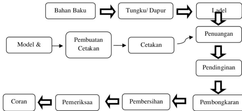
Gambar 1. Diagram Pengecoran
