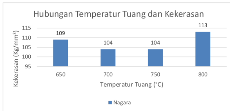
Gambar 13. Hasil Pengujian Kekerasan pada Wajan Nagara
