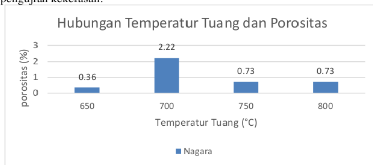
Gambar 12. Hasil Pengujian Porositas pada Wajan Nagara
