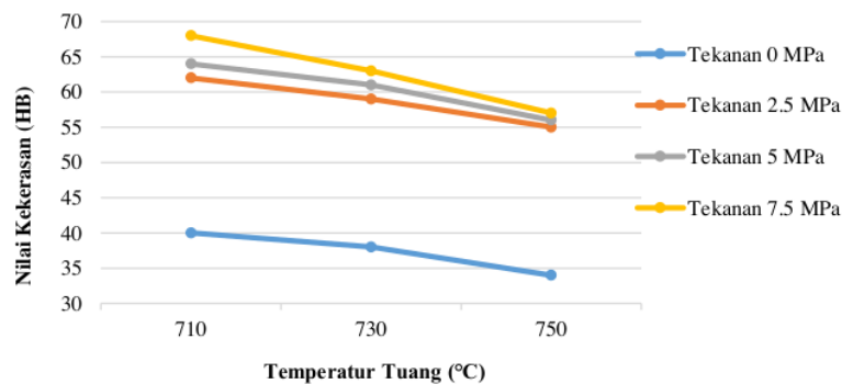
Gambar 2. Grafik hubungan temperatur tuang dan nilai kekerasan pada tekanan (0, 2.5, 5, dan 7.5) MPa.
