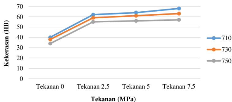
Gambar 3. Grafik hubungan tekanan dan nilai kekerasan pada temperatur tuang (710, 730 dan 750) °C.
