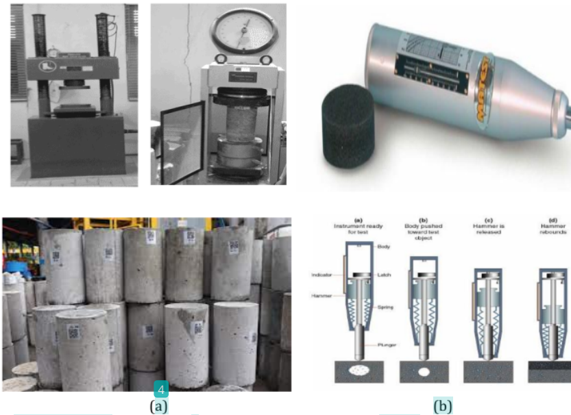
Gambar 4. Alat pengujian: (a). merusak ( destructive test ) dan (b). tidak merusak ( nondestructive test )
