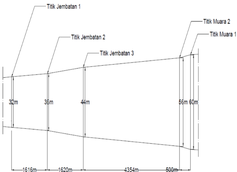
Gambar 2. Skema Pengambilan data titik pada Saluran Primer
