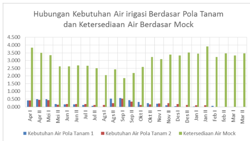
Gambar 3. Grafik Hubungan Ketersediaan Air dan Kebutuhan Air Irigasi
