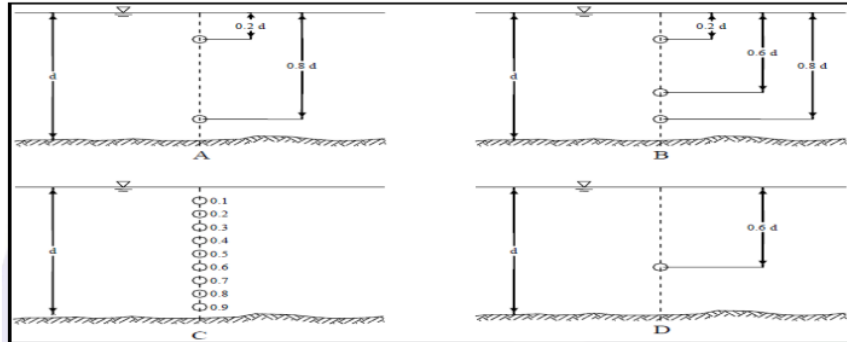
Gambar 1. Pengukuran kecepatan aliran dengan cara 1 titik, 2 titik dan 3 titik
