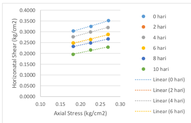
Gambar 6. Hubungan antara Tegangan Aksial dan Horisontal dalam waktu siklus pembersihan untuk kondisi Kekuatan Sisa (Residual)
