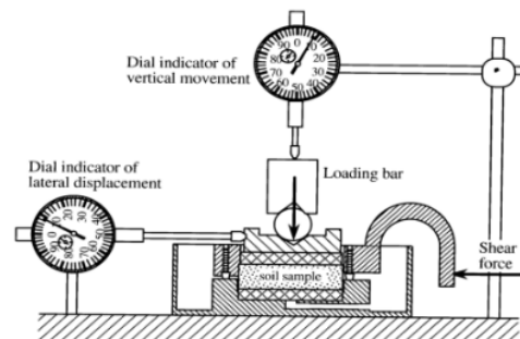
Gambar 1. Skema Alat Uji Geser Langsung
