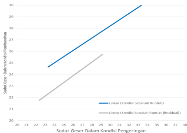
Gambar 9. Hubungan antara Sudut Geser Dalam kondisi pembasahan-pengeringan
