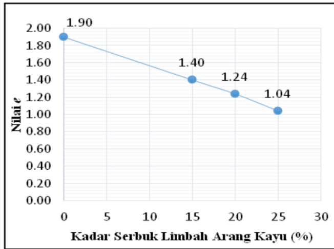
Gambar 3.1 Hubungan Nilai e vs prosentase arang
