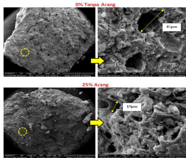
Gambar 3.8 Struktur Mikroskopik Tanah
