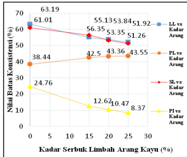
Gambar 3.4 Hubungan Nilai Batas-batas Atterberg vs prosentase arang
