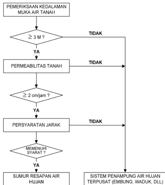
Gambar 2. Diagram alir perencanaan sumur resapan (Suripin, 2004)
