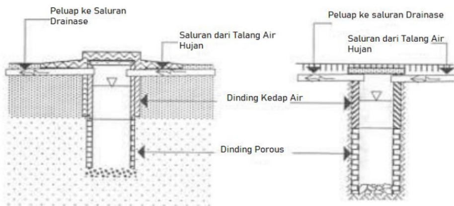
Gambar 2. Detil Konstruksi sumur resapan (Istramaulana, 2014)
