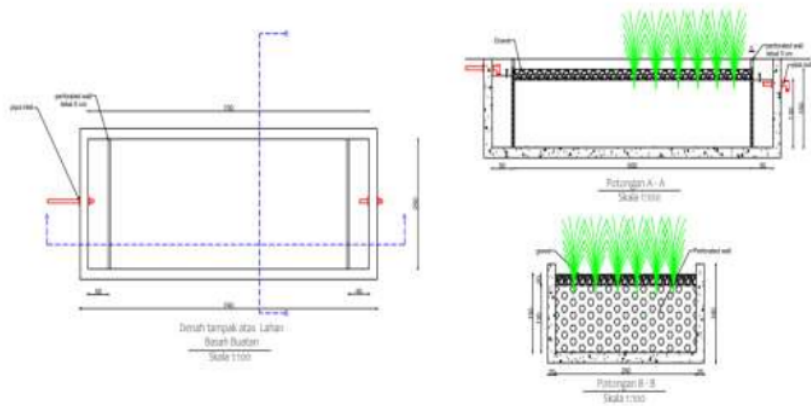
Gambar 5. Desain Lahan Basah Buatan
