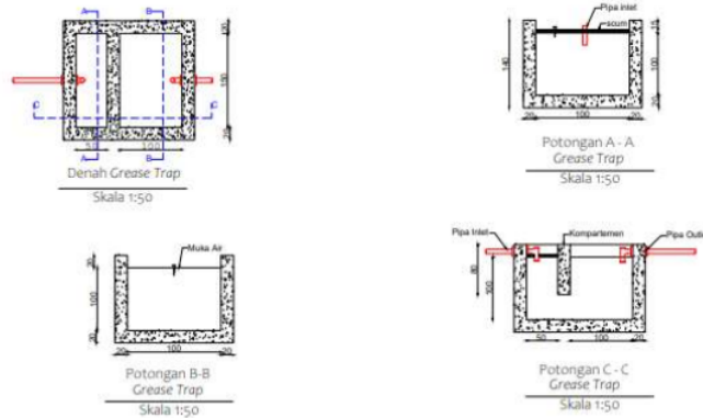
Gambar 2. Desain Grease Trap Rumah Tinggal
