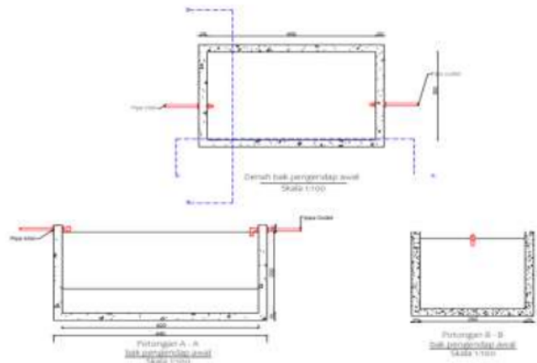
Gambar 3. Desain Bak Pengendap Blok 1
