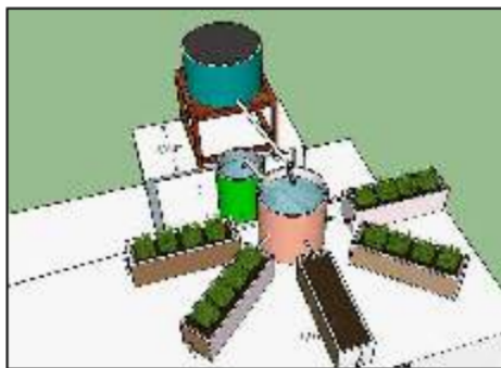
Gambar 1. Desain Reaktor
