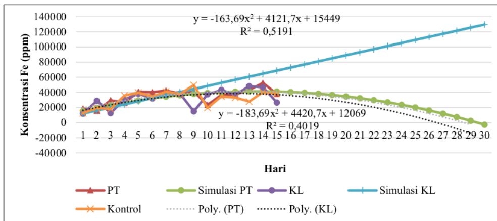
Gambar 9. Simulasi Dinamika Fe pada Purun Tikus dan Kalakalai di Media LBB-AHBP
