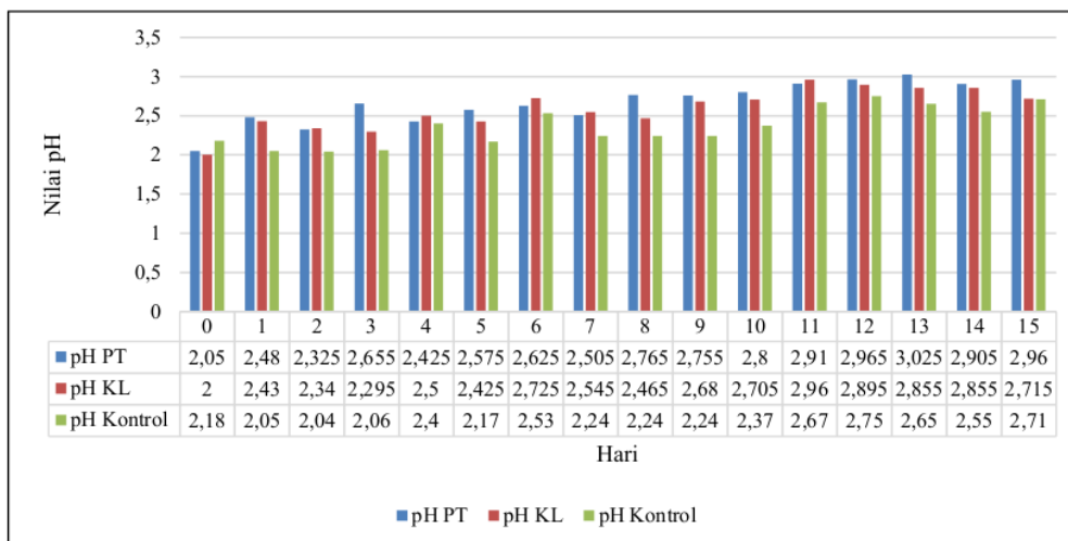
Gambar 2. Nilai pH pada Media Lahan Basah Buatan
