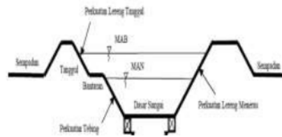
Gambar 1. Penampang Melintang Sungai (Sudaryoko, 1987).
