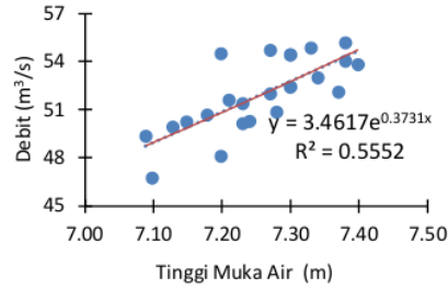
Gambar 8 Lengkung Debit Menggunakan Persamaan Eksponensial
