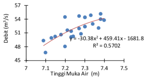
Gambar 6 Lengkung Debit Menggunakan Persamaan Polinomial
