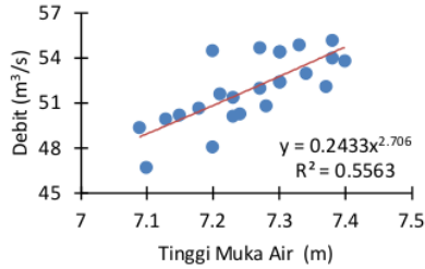
Gambar 7 Lengkung Debit Menggunakan Persamaan Berpangkat ( power )
