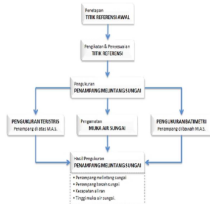
Gambar 3 Bagan Alir Pengukuran Penampang Sungai
