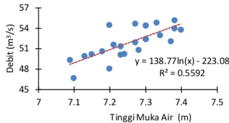
Gambar 5 Lengkung Debit menggunakan Persamaan Logaritmik
