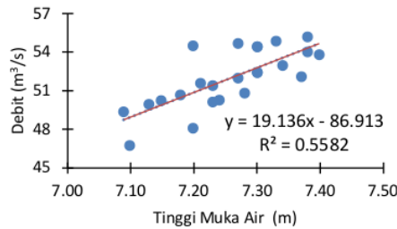
Gambar 4 Lengkung Debit menggunakan Persamaan Linear satu peubah.
