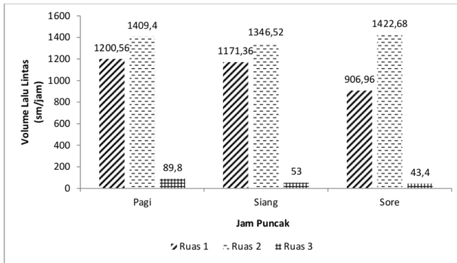
Gambar 3.1 Volume Lalu Lintas di Ketiga Ruas Jalan
