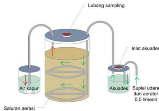
Gambar 1. Desain komposter
