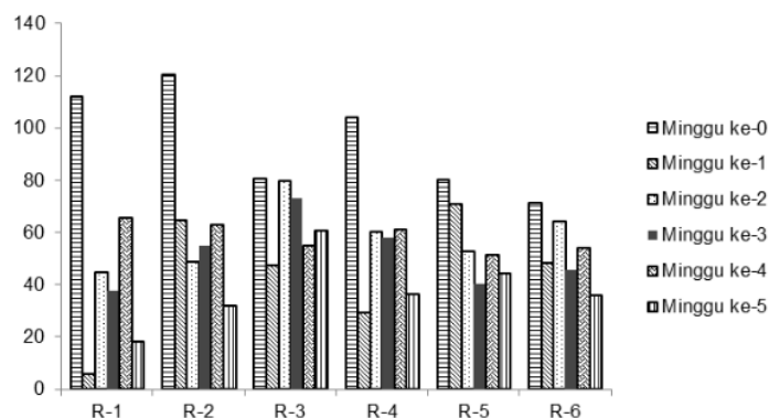
Gambar 4.5. Grafik Hasil Pengukuran Rasio C/N
