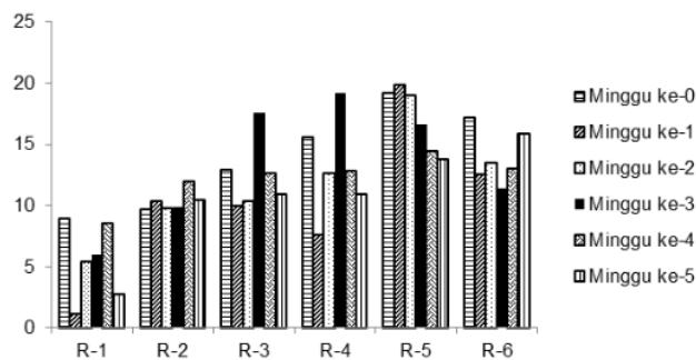
Gambar 3. Hasil Pengujian Kandungan Karbon (C-Organik)
